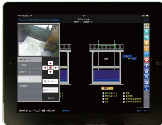
カメラ映像・開度・警報表示 (タブレット端末)
