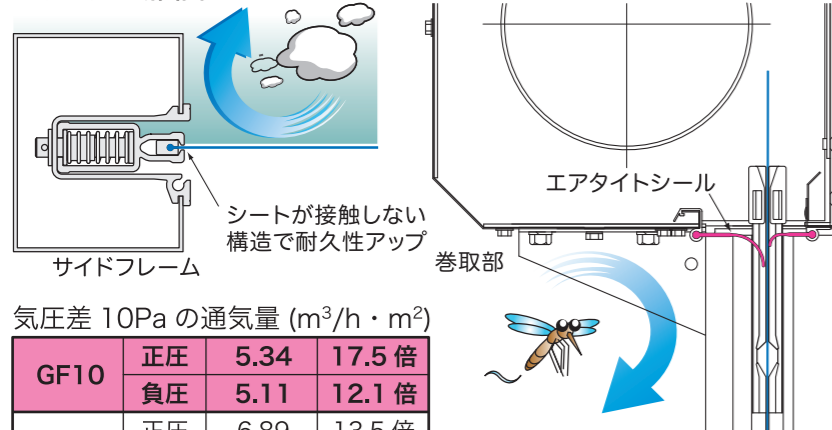
シャッター断面図
