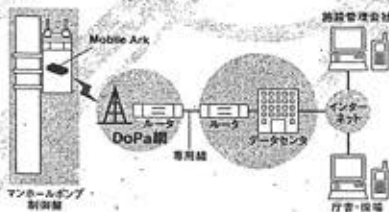
上下水道遠隔監視・制御システム「新水神ネットワーク」イメージ図
