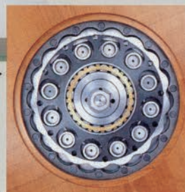
シートシャッター心臓部▶
